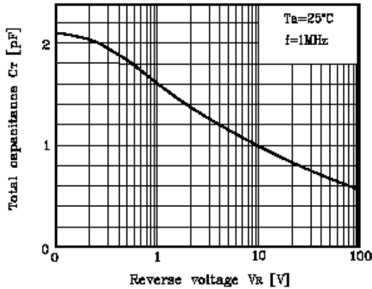
Fig. 3 C_T-V_R
